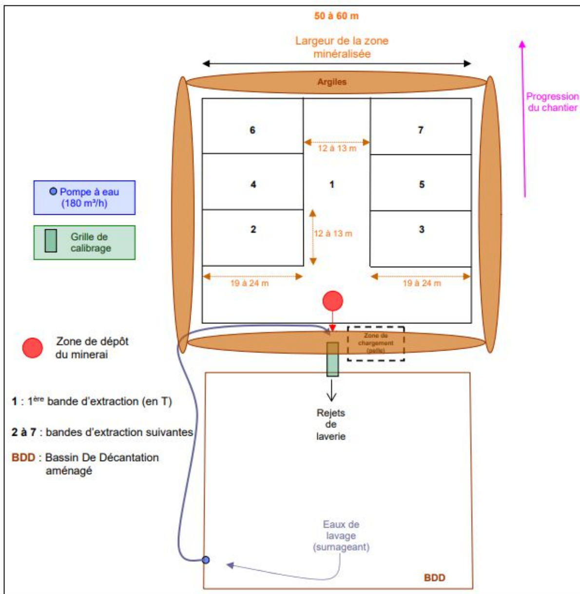
Figure 3 : Schéma de principe de l'exploitation envisagée par la SARL CITE'OR
