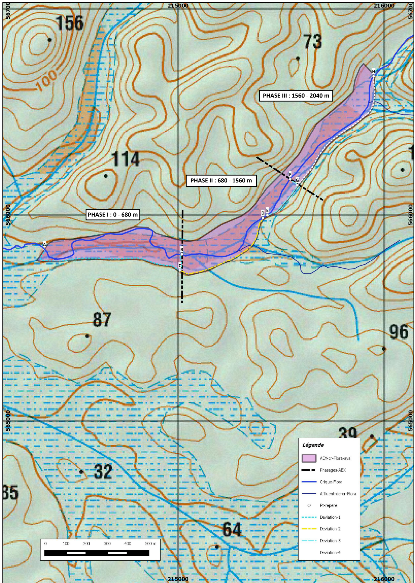
Figure 2 : Situation des dérivations de crique et des phases d'exploitation prévues par la SARL CITE'OR sur un fond IGN adapté au 1/10 000° en UTM22 RGFG95
