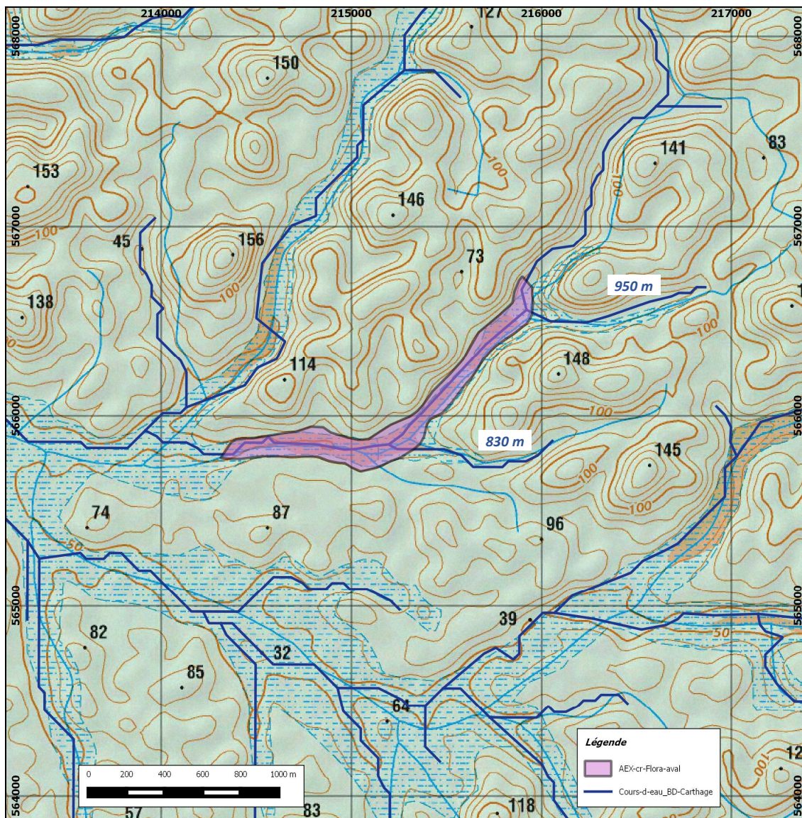
Figure 1 : Situation de l'AEX demandée par la SARL CITE'OR par rapport aux têtes de criques sur un fond de carte IGN au 1/20 000° en UTM22 RGFG95
